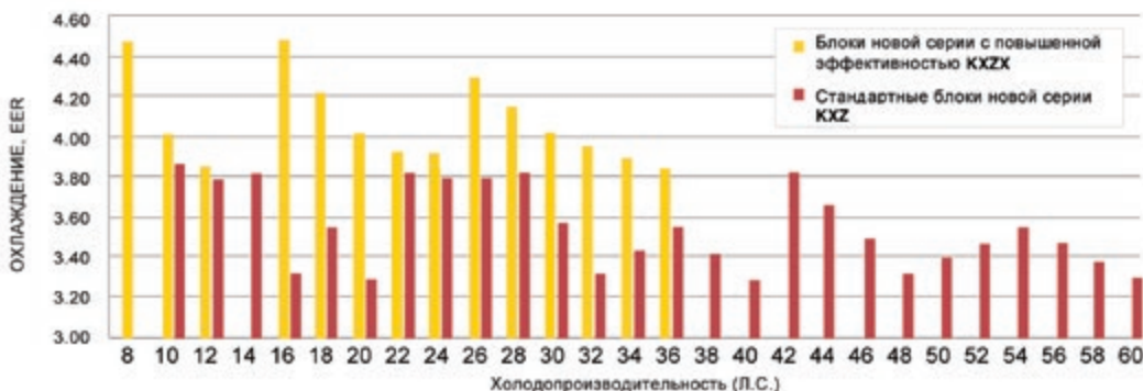
Сравнение коэффициента энергоэффективности стандартных блоков KXZ и блоков с повышенной энергоэффективностью
